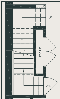
OPTIONAL PANTRY
